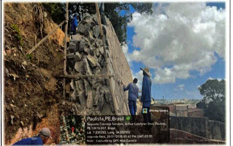
Foto n. 02 EXECUÇÃO DE MURO DE CONTENÇÃO EM PEDRA RACHÃO, COM ASSENTAMENTO EM ARGAMASSA, ENTRE AS ESTACAS E02 E E03.
