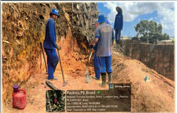
Foto n. 01 ESCAVAÇÃO MANUAL DE VALA COM PROFUNDIDADE MENOR OU IGUAL A 1,30 M, PARA EXECUÇÃO DA BASE DO MURO DE CONTENÇÃO, REFERENTE ÀS ESTACAS E02 E E03.
