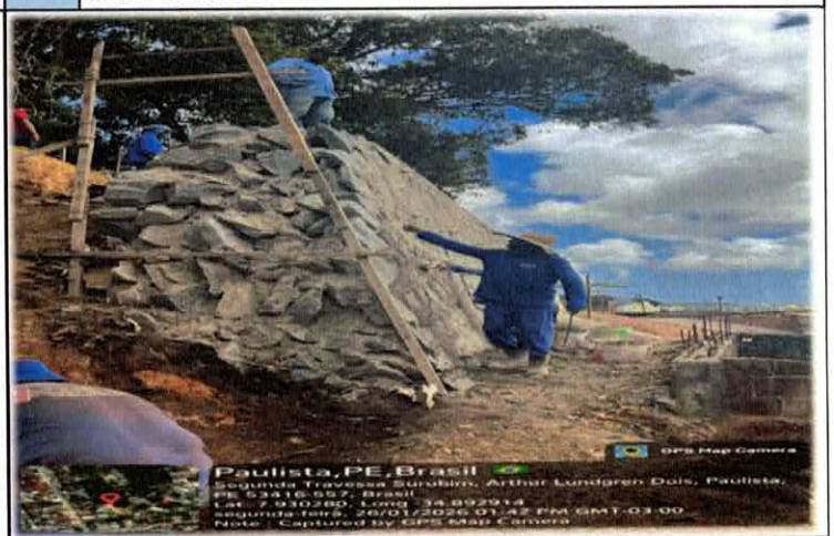
Foto n. 04 EXECUÇÃO DE MURO DE CONTENÇÃO EM PEDRA RACHÃO, COM ASSENTAMENTO EM ARGAMASSA, ENTRE AS ESTACAS E02 E E03.
