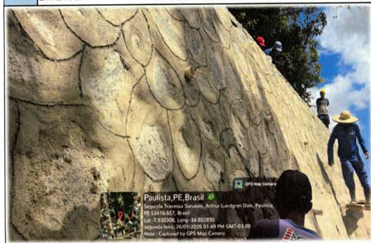
Foto n. 05 INSTALAÇÃO DE TUBO DE ESGOTO, COM CAMADA DE BRITA E BIDIM, PARA ESCOAMENTO (DRENAGEM) DE ÁGUAS PLUVIAIS.
