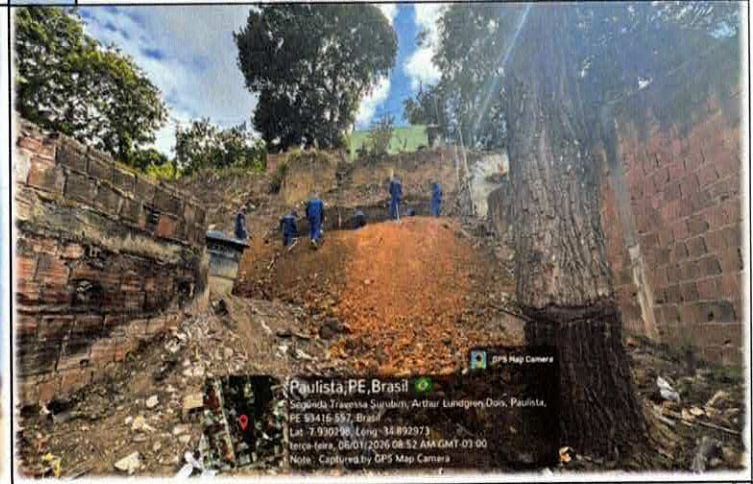
Foto n. 06 ESCAVAÇÃO MANUAL DE VALA COM PROFUNDIDADE MENOR OU IGUAL A 1,30 M, PARA EXECUÇÃO DA BASE DO MURO DE CONTENÇÃO, REFERENTE ÀS ESTACAS E02 E E03.
