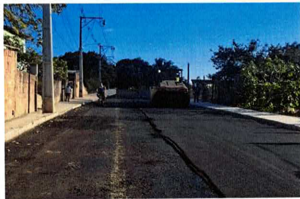
5.8 - EXECUÇÃO DE PAVIMENTO COM APLICAÇÃO DE CONCRETO ASFÁLTICO
