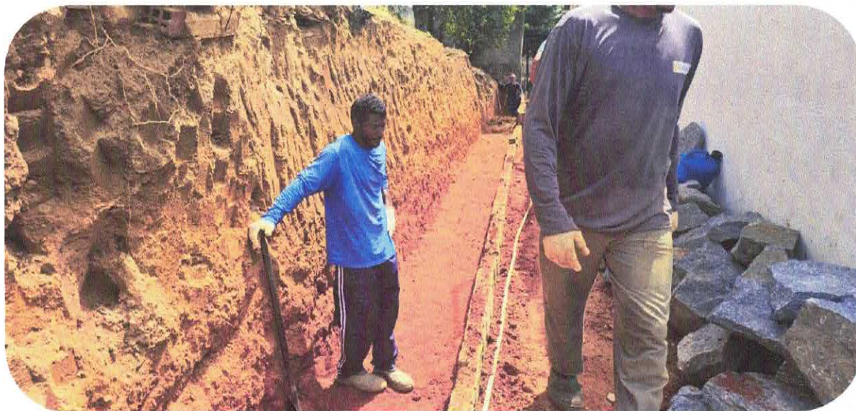
3.1.3. REGULARIZAÇÃO E COMPACTAÇÃO DE TERRENO, COM SOQUETE - (OBRA 02).
