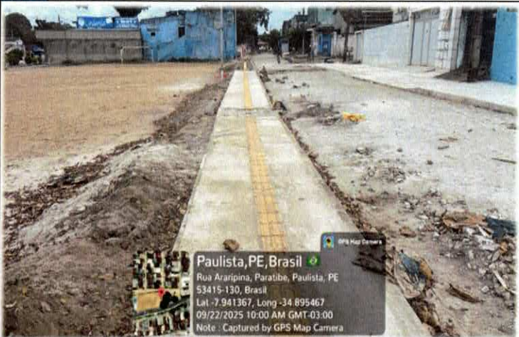
Foto n. 12 EXECUÇÃO DE PASSEIO EM LADRILHO HIDRÁULICO TÁTIL ALERTA AMARELO APLICADO SOBRE LASTRO DE CONCRETO.
