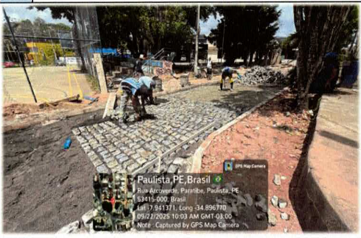
Foto n. 03 PAVIMENTO EM PARALELEPÍPEDO SOBRE COLCHÃO DE AREIA REJUNTADO COM ARGAMASSA DE CIMENTO.
