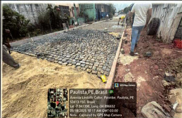
Foto n. 10 PAVIMENTO EM PARALELEPÍPEDO SOBRE COLCHÃO DE AREIA.
