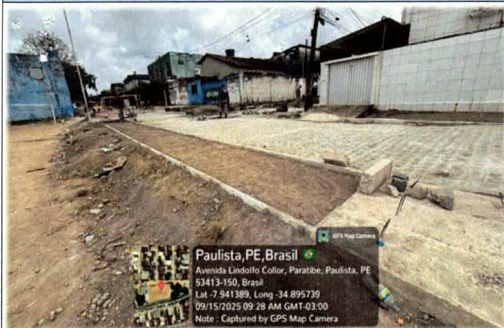
Foto n. 07 REGULARIZAÇÃO MANUAL DE TERRENO NATURAL COM CORTE OU ATERRO.
