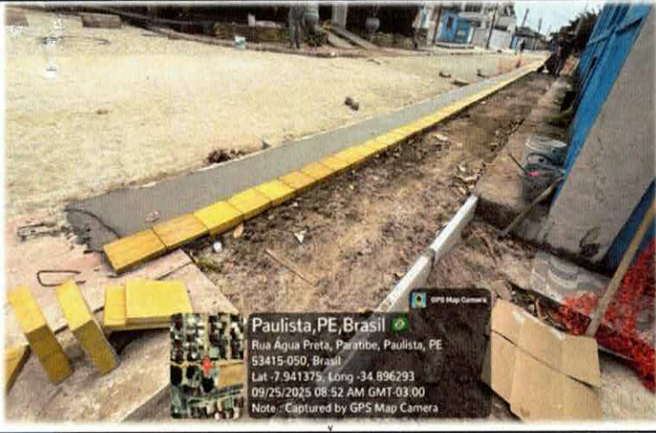
Foto n. 01 EXECUÇÃO DE PASSEIO EM LADRILHO HIDRAULICO TATIL AMARELO.
