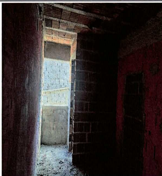
FOTO 09: 3.4.0.0.1. ALVENARIA EM TIJOLO CERAMICO FURADO, 1/2 VEZ, ASSENTADO EM ARGAMASSA TRACO 1:4 (CIMENTO E AREIA MEDIA NAO PENEIRADA), PREPARO MANUAL, JUNTA 1 CM
