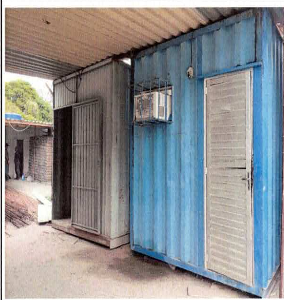
FOTO 20: EXECUÇÃO DE ESCRITÓRIO EM CANTEIRO DE OBRA EM ALVENARIA, NÃO INCLUSO MOBILIÁRIO E EQUIPAMENTOS. AF_02/2016
