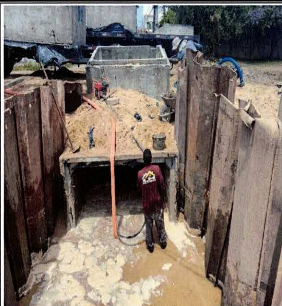
FOTO 12: 5.2.0.0.4. ESGOTAMENTO COM BOMBA CENTRÍFUGA MONOESTÁGIO COM MOTOR ELÉTRICO O A COMBUSTÃO CHP DIURNO
