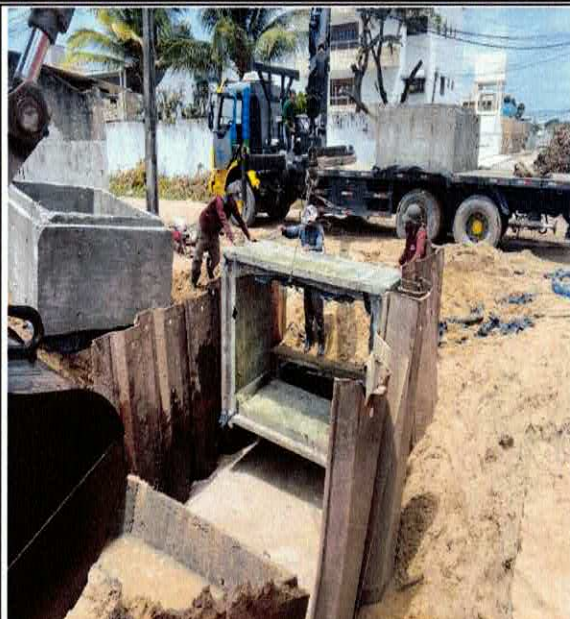
FOTO 16: ASSENTAMENTO DE ADUELAS PREMOLDADAS EM CONCRETO ARMADO SEÇÃO 2,2 X 1,5
