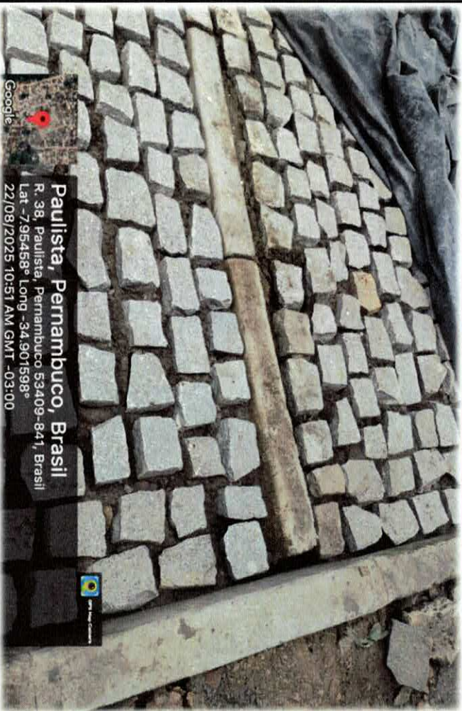
Foto n. 09 MEIO-FIO EM PEDRA GRANITICA
