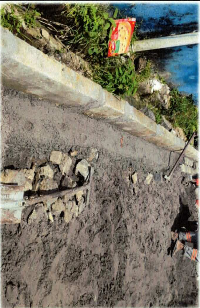
Foto n. 05 LINHA D'ÁGUA COM PARALELEPÍPEDOS GRANÍTICOS
