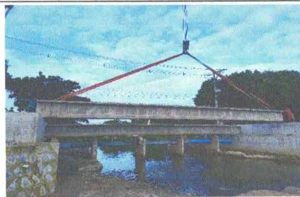
9.2.10 - Lançamento de viga pré-moldada com utilização de guindaste
