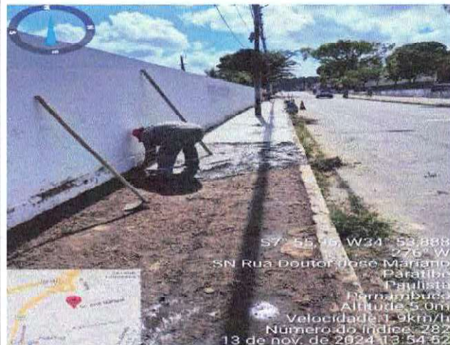
EXECUÇÃO DE CALÇADA – RUA DR JOSÉ MARIANO, PARATIBE – PAULISTA/PE
