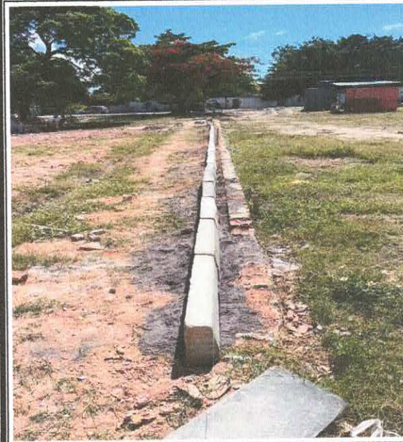
Foto 16: 7.1.0.4. Assentamento de guia (meio-fio) em trecho reto ou curvo. (01/01/24 a 10/02/24)
